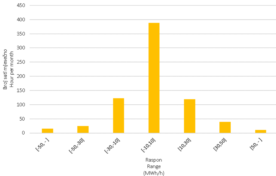
Slika 10 Statistička raspodjela satnih promjena proizvodnje VE u rujnu 2019. godine Figure 10 Statistical distribution of WPP hourly output variations in September 2019
