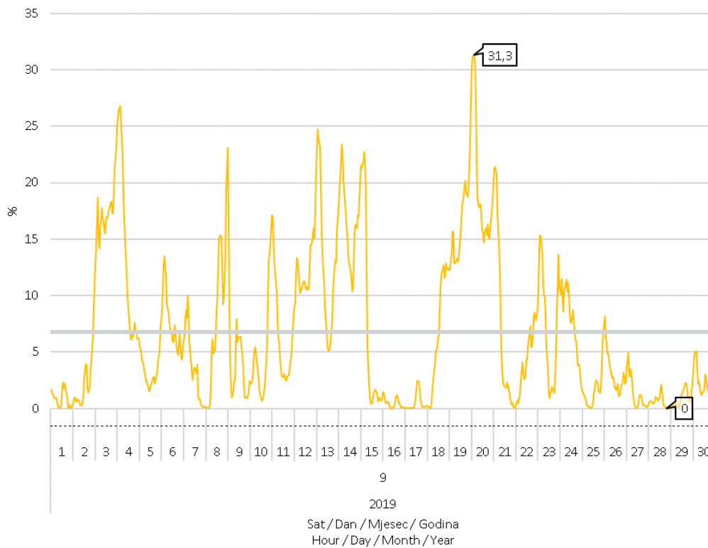
Slika 8 Udio proizvodnje vjetroelektrana u pokrivanju satnog opterećenja elektroenergetskog sustava u rujnu 2019. godine
