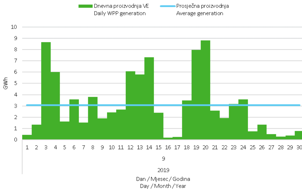
Slika 5 Dnevna proizvodnja svih vjetroelektrana u rujnu 2019. godine
