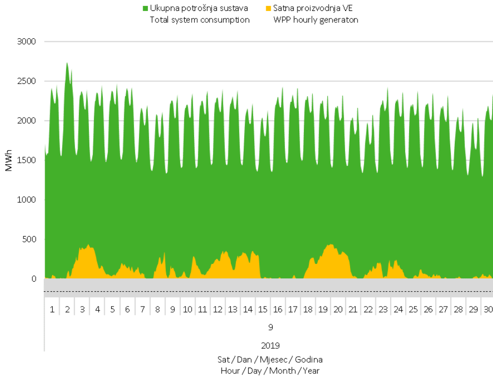
Slika 7 Usporedba satnog dijagrama opterećenja sustava i proizvodnje vjetroelektrana u rujnu 2019. godine
