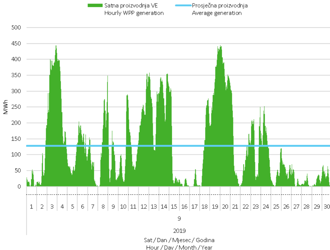
Slika 2 Satna proizvodnja svih vjetroelektrana u rujnu 2019. godine
