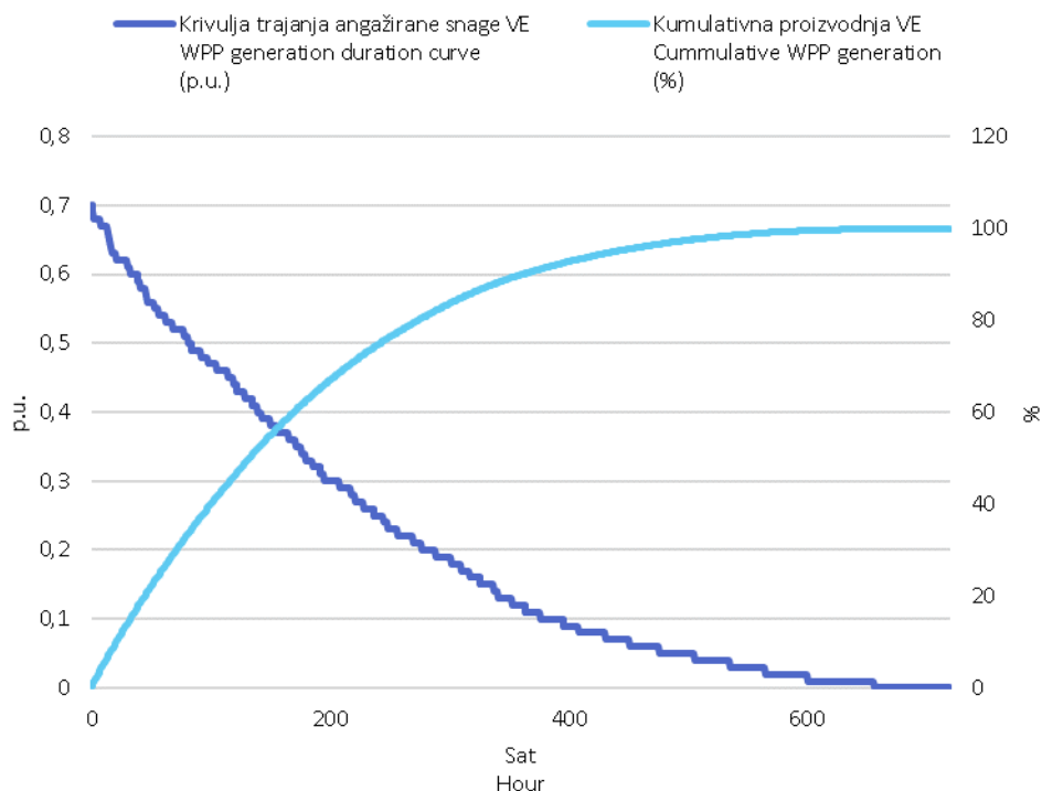
Slika 3 Krivulja trajanja angažirane snage svih VE i kumulativna proizvodnja VE u rujnu 2019. godine u jediničnim vrijednostima
