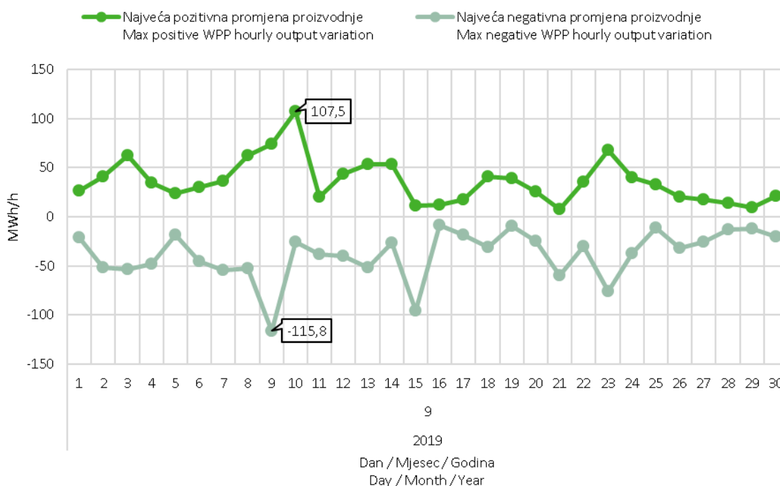
Slika 9 Maksimalna pozitivna i maksimalna negativna promjena satne proizvodnje VE u rujnu 2019. godine
