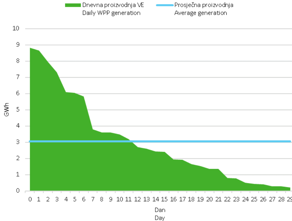
Slika 6 Krivulja trajanja dnevne proizvodnje vjetroelektrana u rujnu 2019. godine
